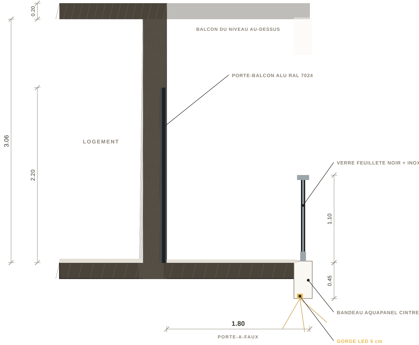
3 · COUPE B-B — AU PETIT LOBE · 1:25
