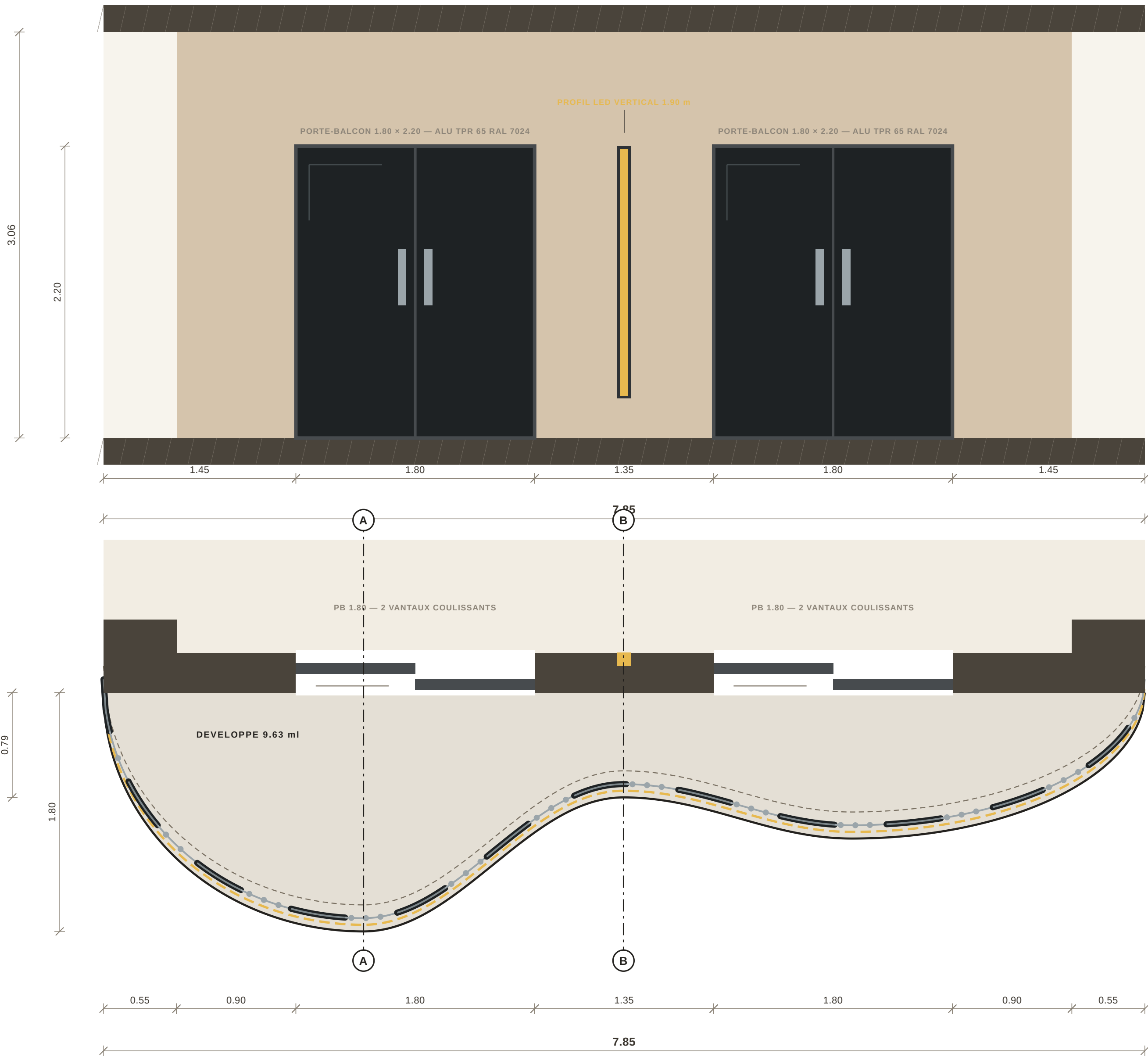
1 · ELEVATION INTERIEURE DU BALCON · 1:25
